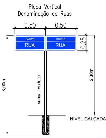
Detalhe da Sinalização Vertical
