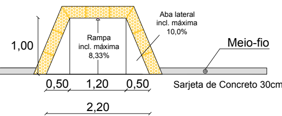
Detalhe Rampa Tipo 01 e Piso Tátil
